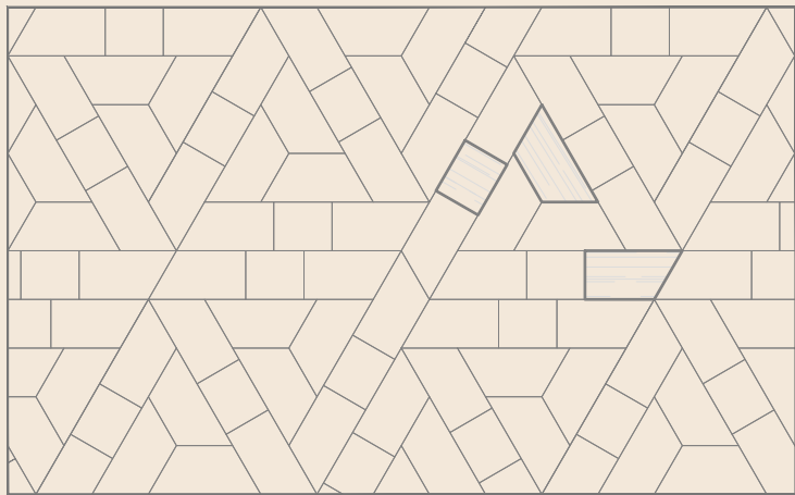
Frato 462x200mm, 400x200mm, 239x200mm
